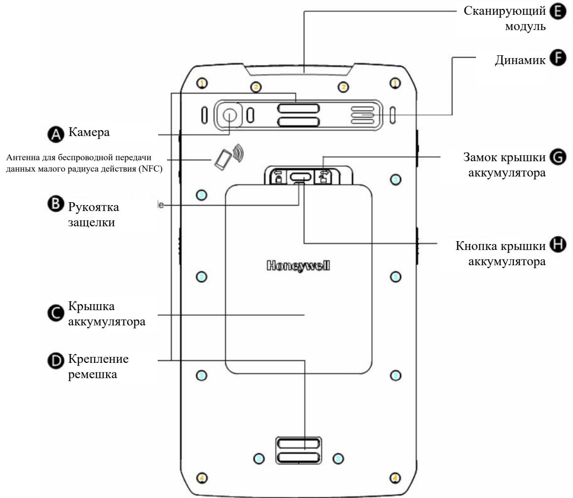
Вид EDA70-X сзади
